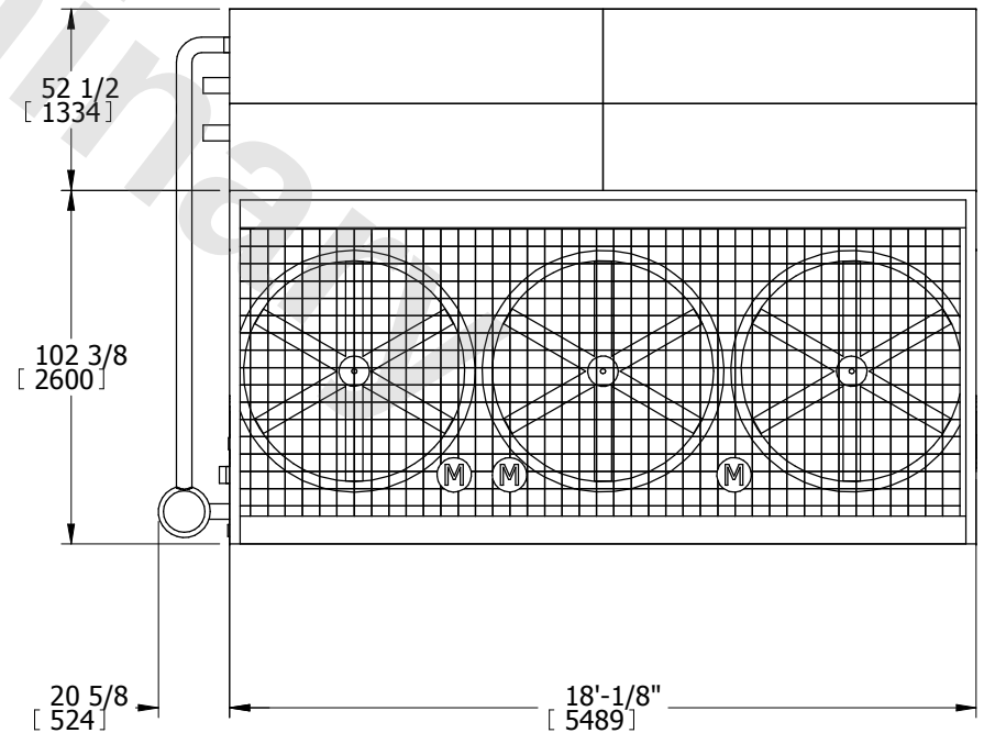
FACE 2
