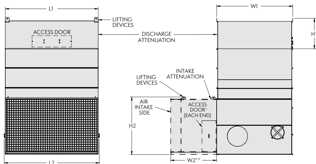
eco-LSWE Attenuation
