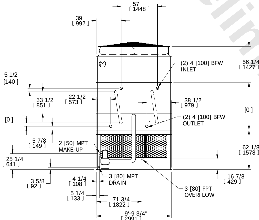
FACE 2
