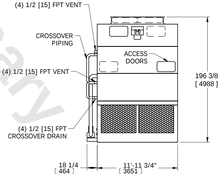
FACE 1
