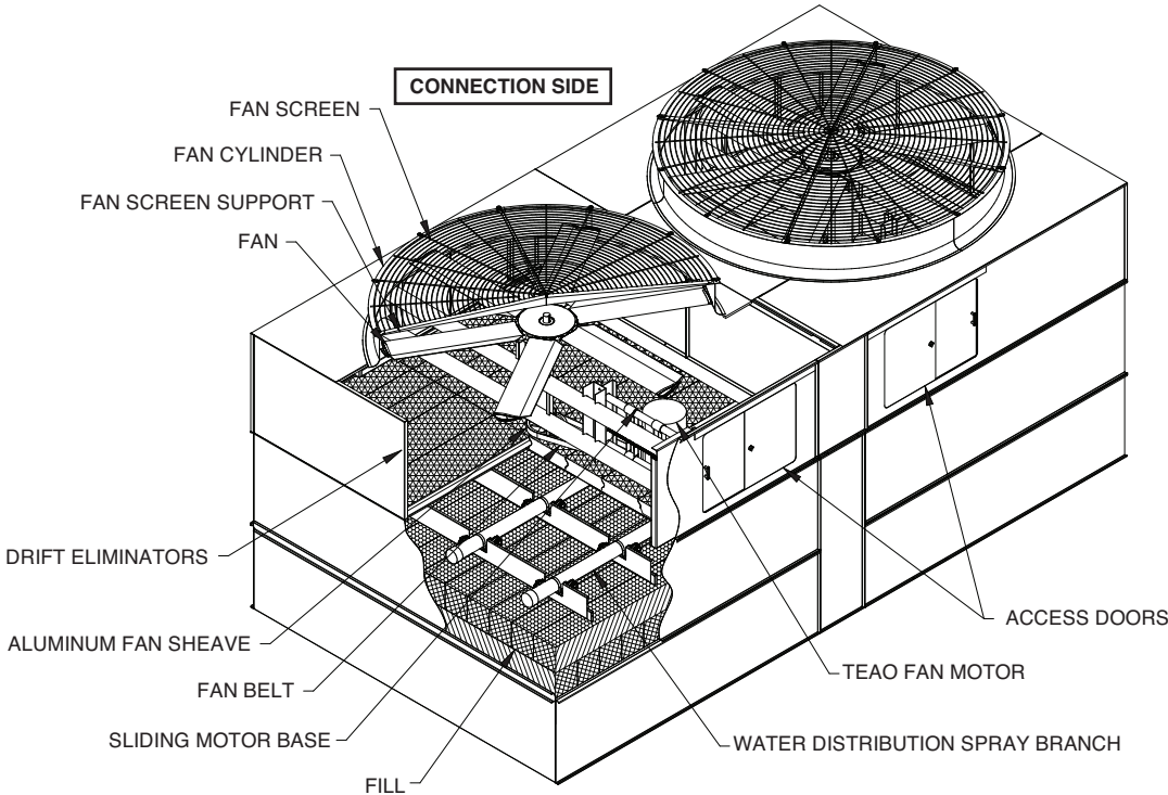
FAN & FILL CASING SECTION
