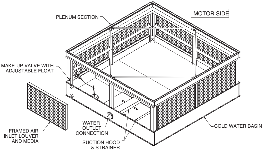
PAN & PLENUM SECTION
