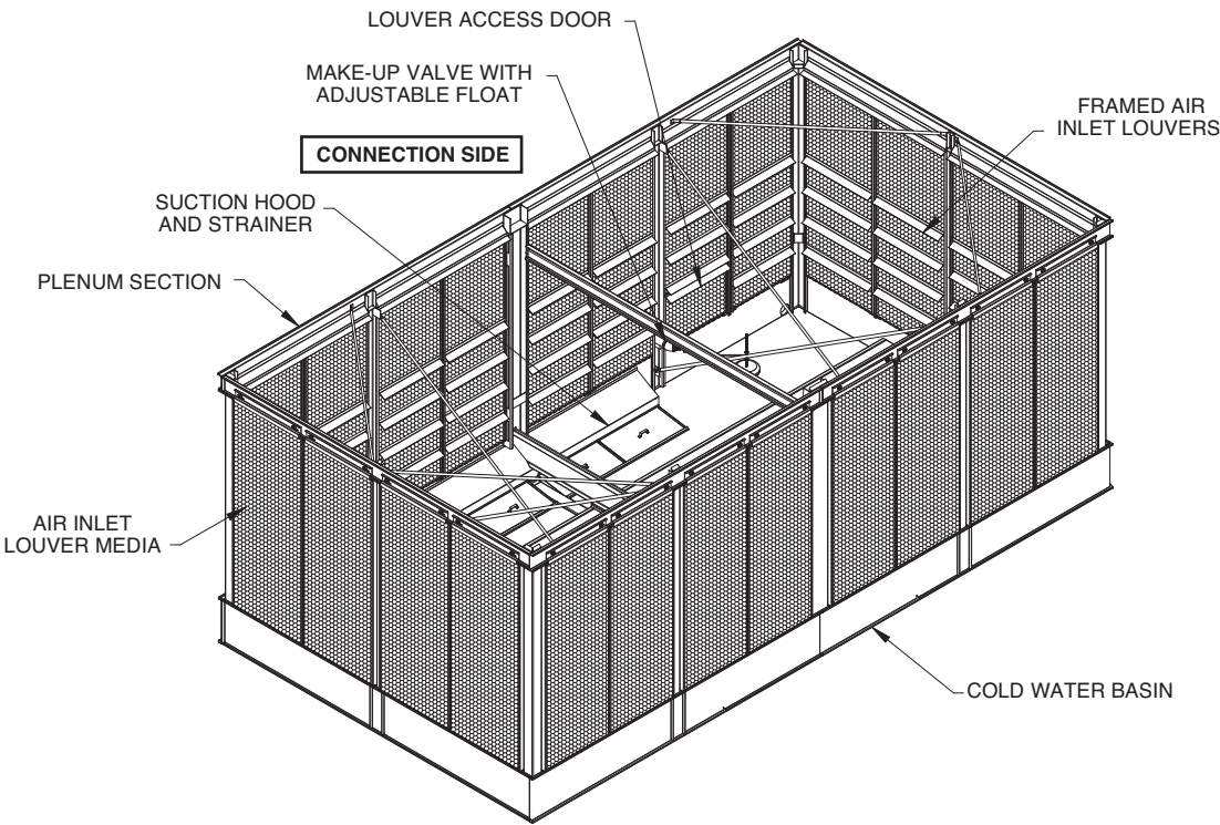
PAN & PLENUM SECTION
